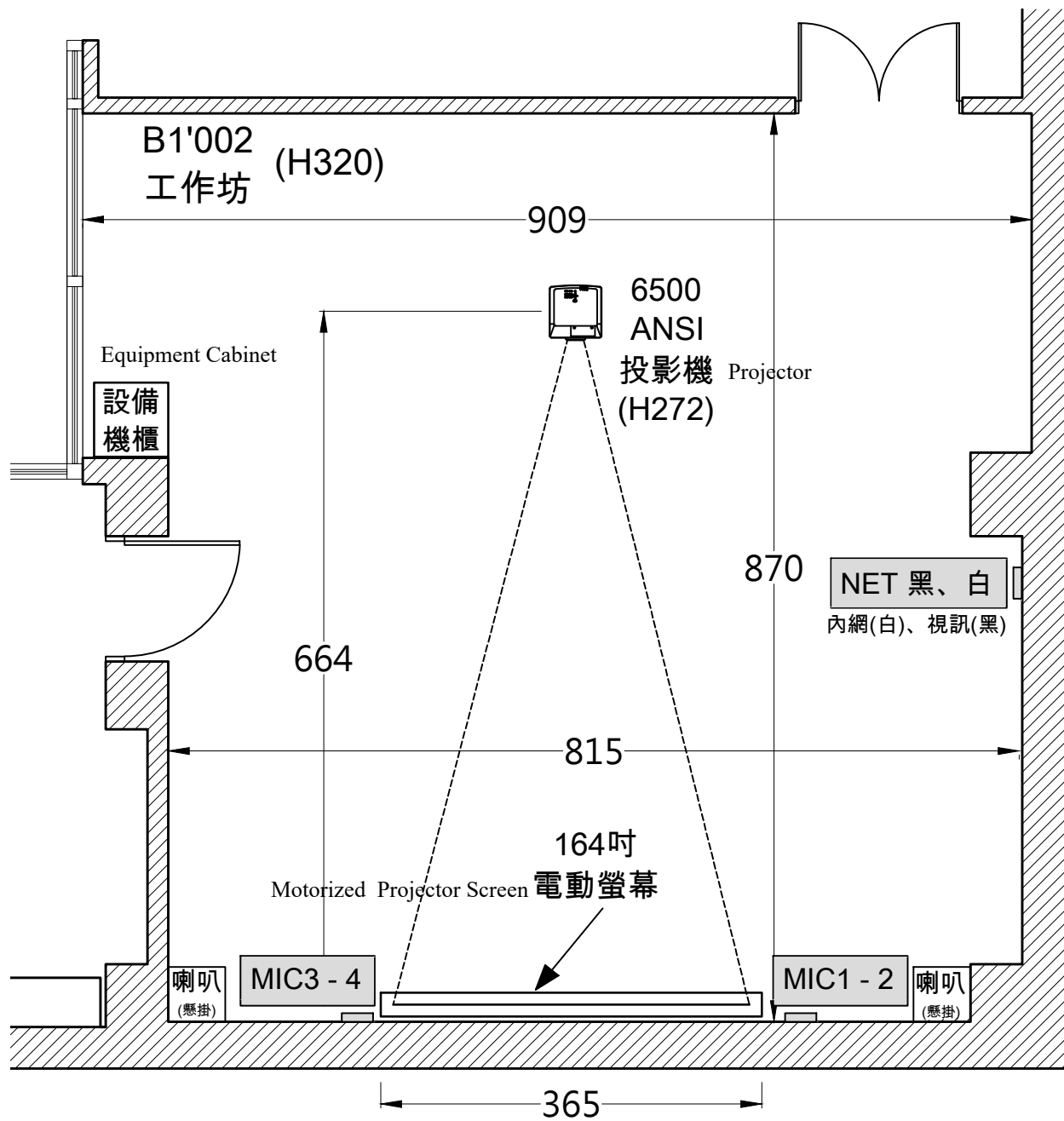
圖 (二) 臺音館工作坊__空間尺寸及音響視訊配置圖 (單位：公分) Figure(2) Workshop__Floor Plan and Audio & Video Plan (Unit: cm)
